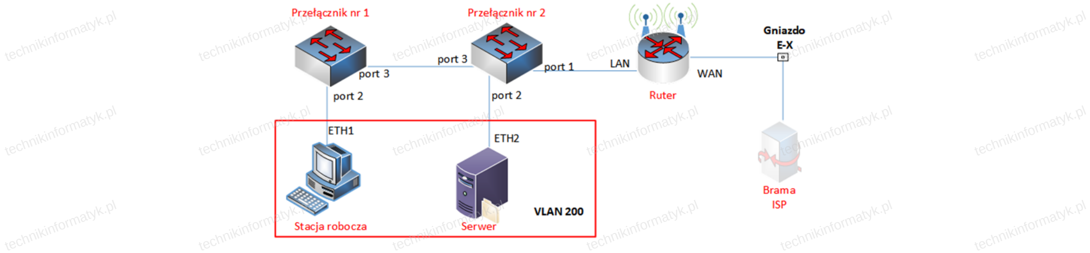
Rys. Schemat połączenia urządzeń sieciowych
