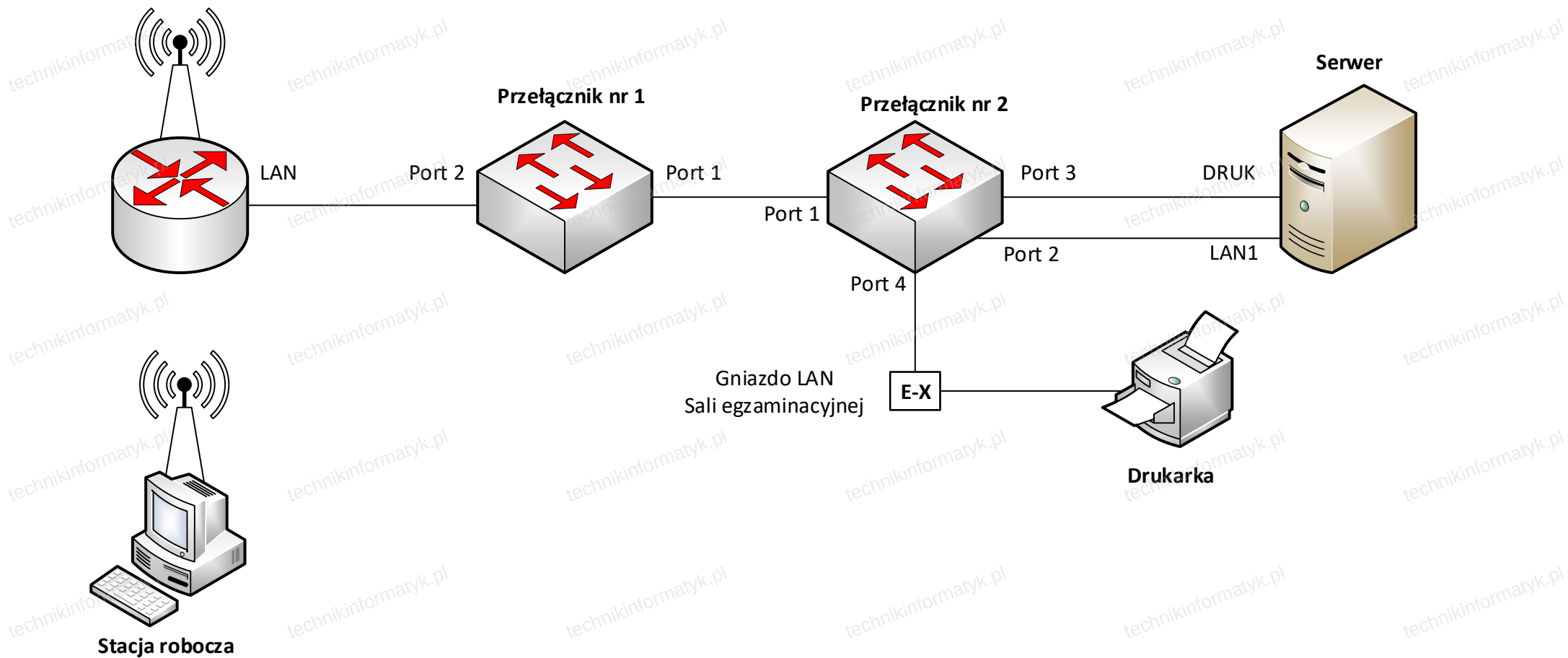
Schemat połączenia urządzeń sieciowych
