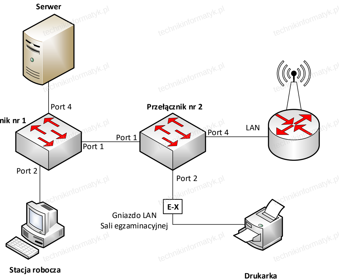
Schemat połączenia urządzeń sieciowych
