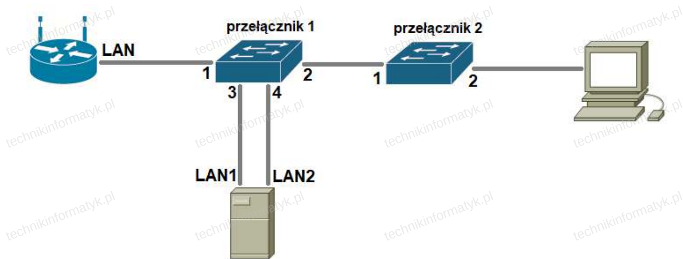
Schemat połączenia urządzeń sieciowych
