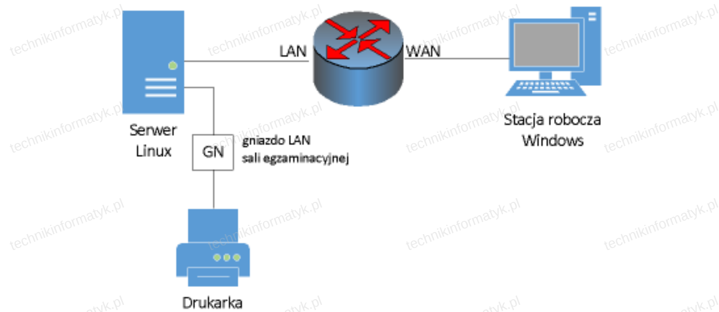
Schemat połączenia urządzeń sieciowych
