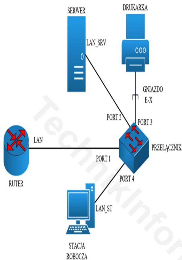
Załącznik 1. Schemat połączenia urządzeń
